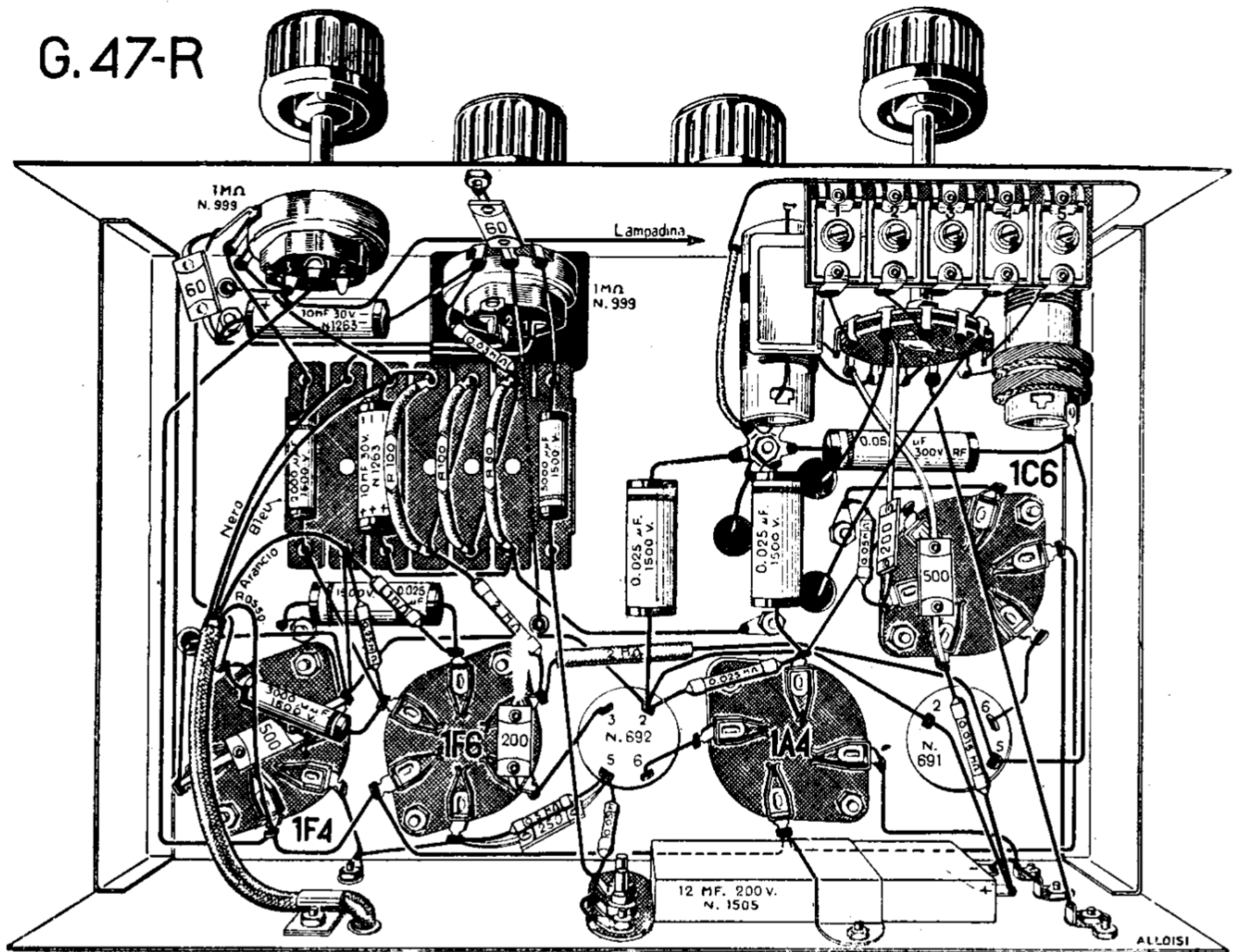
Piano di costruzione.
